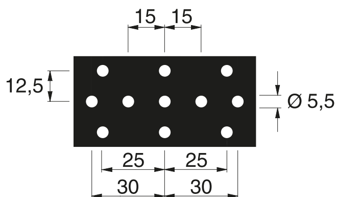
Panou RL cu găuri rotunde
