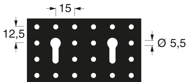
Panou SL cu găuri rotunde și cheie, combinate
